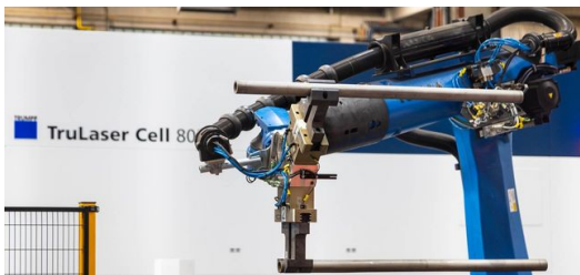
<p>TruLaser Cell 8030
