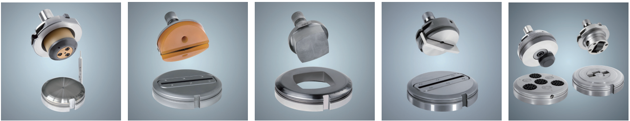
TRUMPF의 다양한 펀칭 틀
