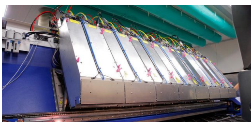
Die Boxen mit den Optiken sind in einer Brücke untergebracht, die die Förderstrecke überspannt. Bild: Ralf Kreuels
