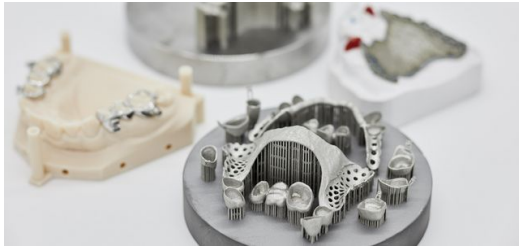
<p>Zahnersatz aus dem 3D-Drucker TruPrint 1000 von TRUMPF.</p>
