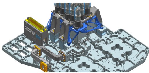
<p>Im Auftrag von Tesat-Spaceroom.com hat TRUMPF eine Halterung für den Kommunikationssatelliten Heinrich Hertz mit 3D-Druck optimiert (im Bild blau markiert) und dabei 55 Prozent Gewicht gespart. </p>
