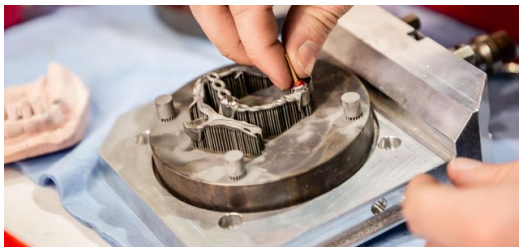
<p>In der TruPrint 1000 wird die Teleskopkrone aus dem Pulverbett aufgebaut. Die Kronen sind bis auf ein minimales Übermaß an den Innenseiten schon nahezu perfekt an die Geometrie des Primärteiles angepasst. (Bild: Steffen Müller-Klenk)</p>
